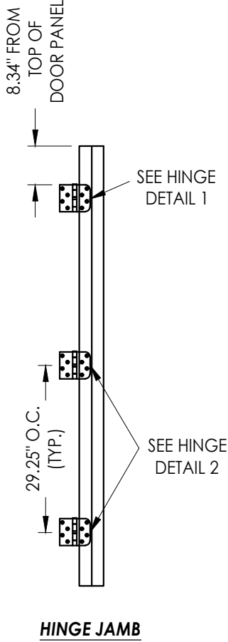
HINGE JAMB
